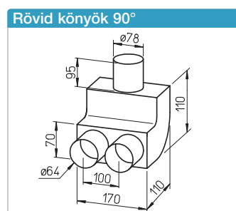
Rövid könyök 90°
